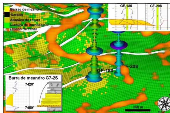
Figura 18. Vista en perspectiva de los pozos GF-180 y GF-208 integrando el modelado de facies (geomodelo) y el cubo de amplitud sísmica con opacidad de amplitudes positivas para la unidad G7-2S. La imagen en la esquina inferior izquierda muestra la descripción del núcleo y su correspondiente registro (GR), con el desarrollo de una barra de meandro. La imagen en la esquina superior derecha muestra la correlación interpretada entre los pozos GF-180 y GF-208, donde el primero atraviesa un cuerpo arenoso (celdas en amarillo en el geomodelo) interpretado como barras de meandro y el segundo pozo atraviesa depósitos lutíticos correspondientes al posible relleno y abandono del canal. Fuente: Modificado de RODRÍGUEZ et al. (2013).
