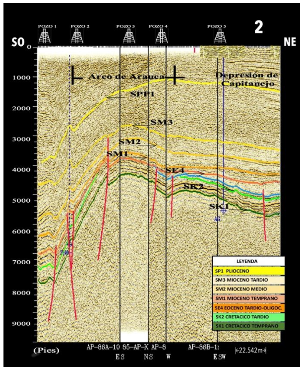
Figura 2. Línea sísmica SO-NE (ubicación en Figura 1A), donde se observa la estratigrafía interpretada y el alto estructural correspondiente al Arco de Arauca.
