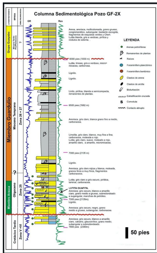
Figura 6. Columna sedimentológica y registro del pozo GF-2X (Holoestratotipo de la Formación Guafita). Fuente: Modificado de ORTEGA et al. (1987).
